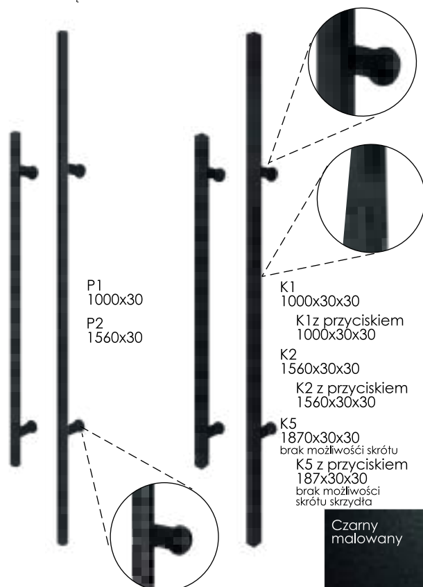
POCHWYT OKRĄGŁY
