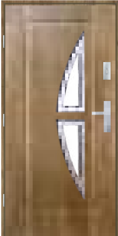
Wzór 10s2
