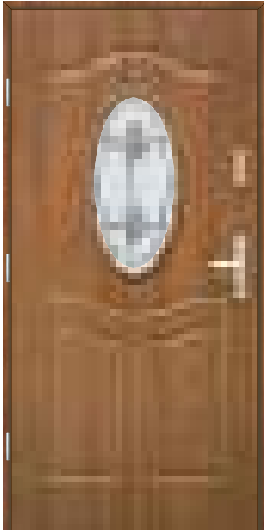
Wzór 6s
