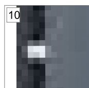
10 6 bolców antywyważeniowych
