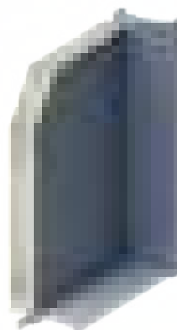
54 PRZECIWOŻAROWE (wewnętrzne)
