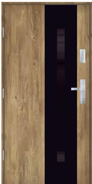
Wzór Perfekt 9
