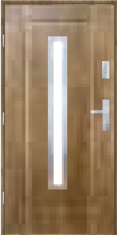
Wzór 10s1
