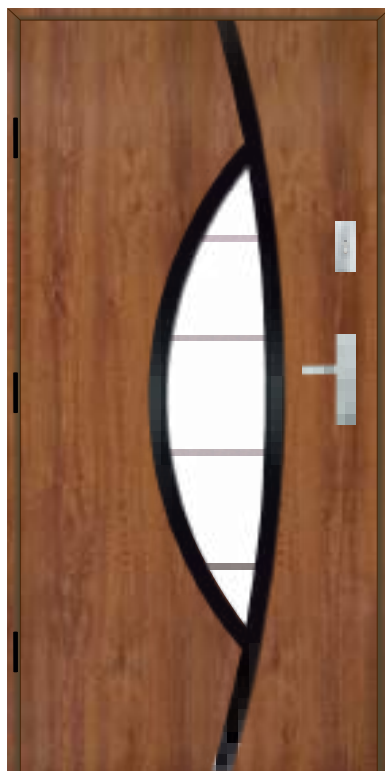
Wzór 11s6
