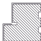
Drewniano-stalowa DS”L”/54
