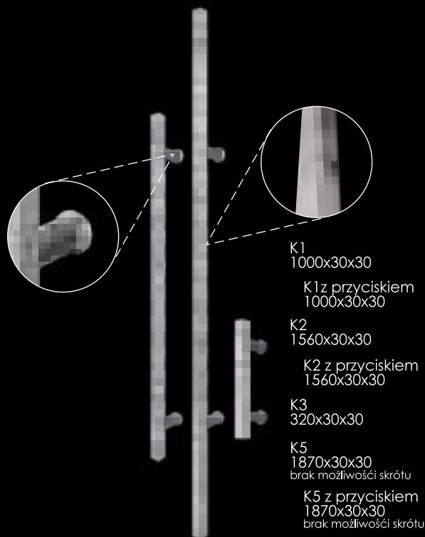
POCHWYT KWADRATOWY
