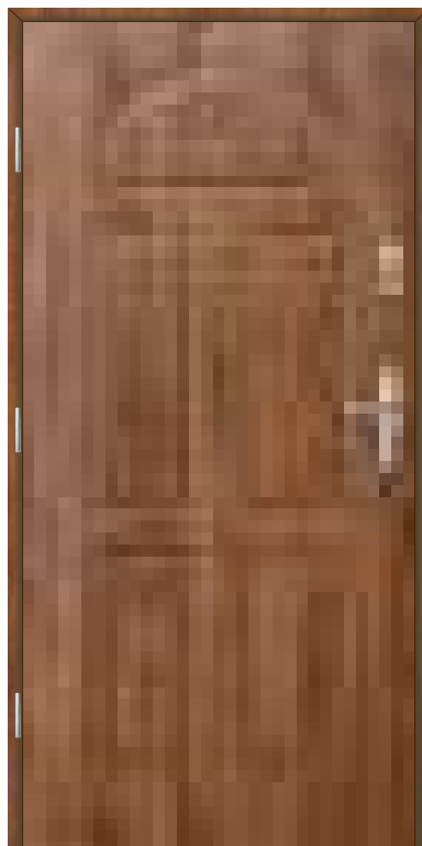
Wzór 2
