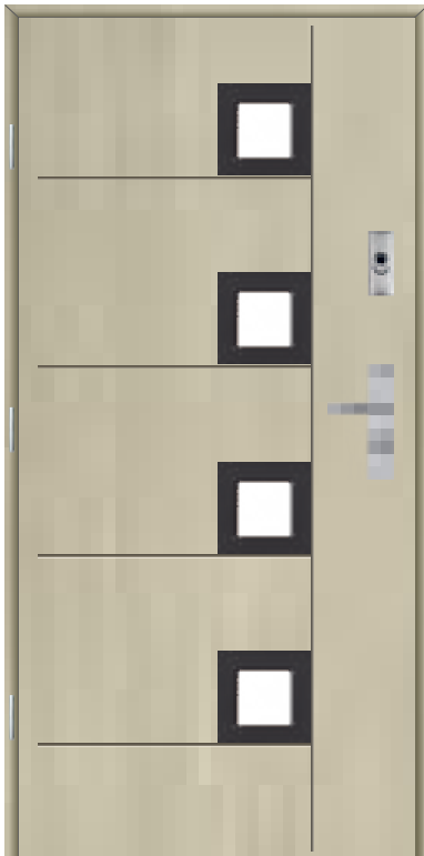
Wzór 14s1
