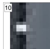
10 3 bolce antywyważeniowe
