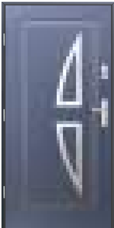
Aplikacja 10-2
