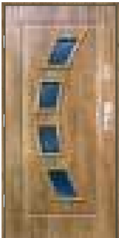
Wzór 10s5
