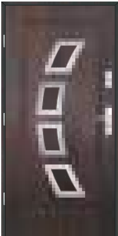
Aplikacja 10-5
